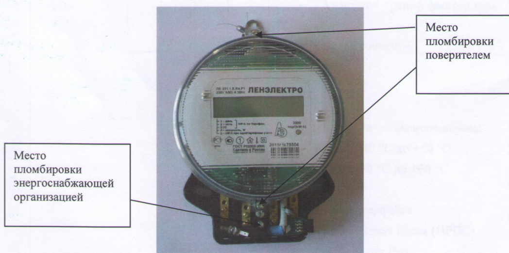
Рисунок 2 - Общий вид счетчика в корпусе ЛЕ.....РО или Р1
