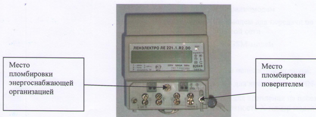
Рисунок 3 - Общий вид счетчика в корпусе ЛЕ.....Д0...
