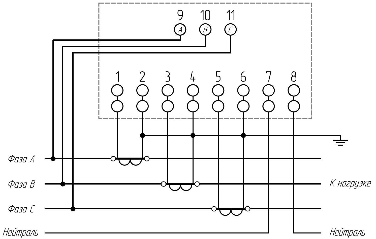
Схема подключения к сети счетчиков электрической энергии трехфазных многотарифных ЛЕ-3 трансформаторного включения
