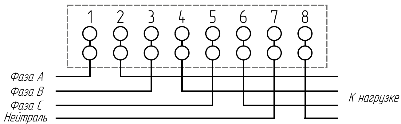
Схема подключения к сети счетчиков электрической энергии трехфазных многотарифных ЛЕ-3 прямого включения
