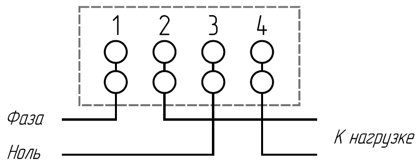
Схема подключения к сети счетчиков электрической энергии однофазных ЛЕ-2
