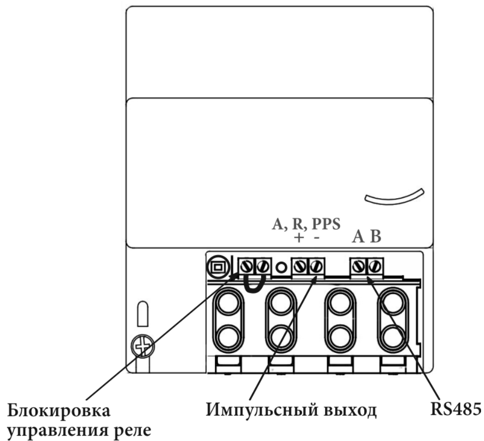
Интерфейсы счетчиков ЛЕ-2 модели D5 без переключателя управления реле
