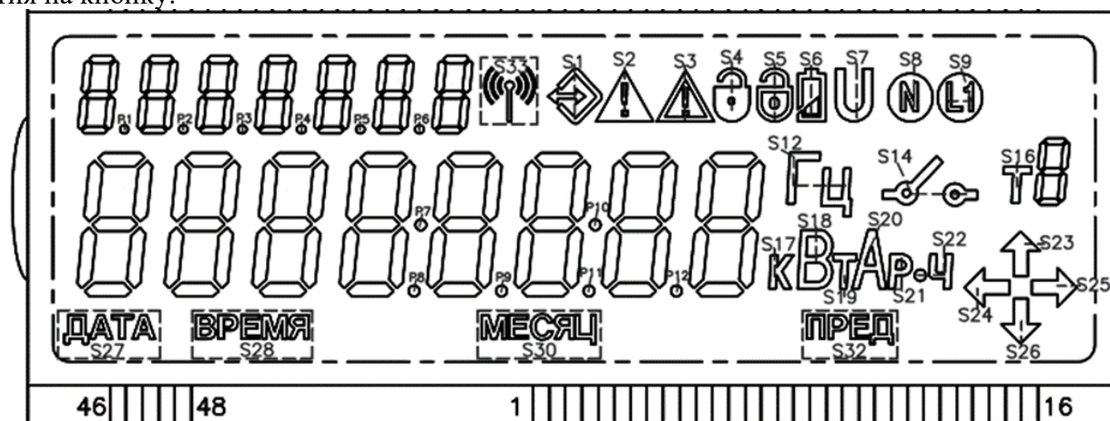
Рисунок 8. Расположение информации на индикаторе
