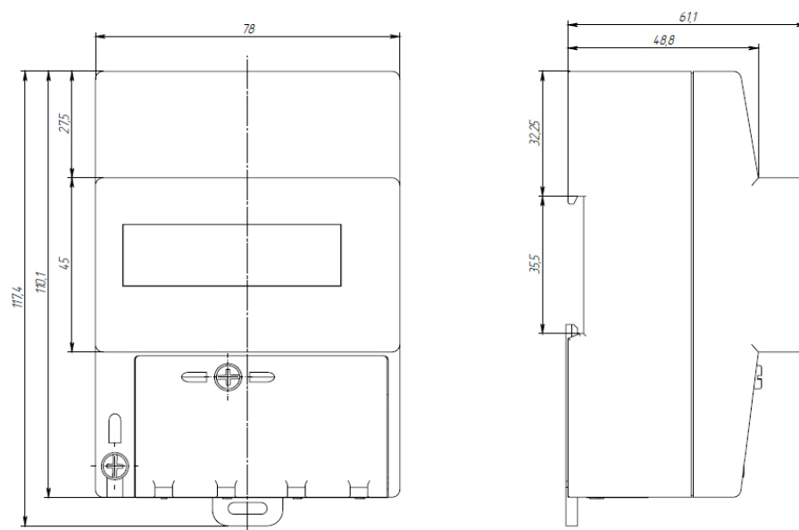
Внешний вид счетчиков
