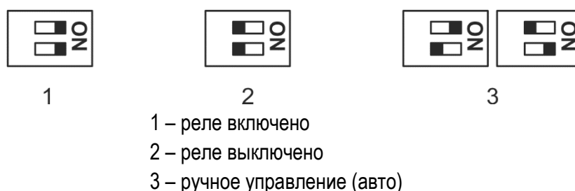
Рисунок 7. Переключение режимов управления реле
