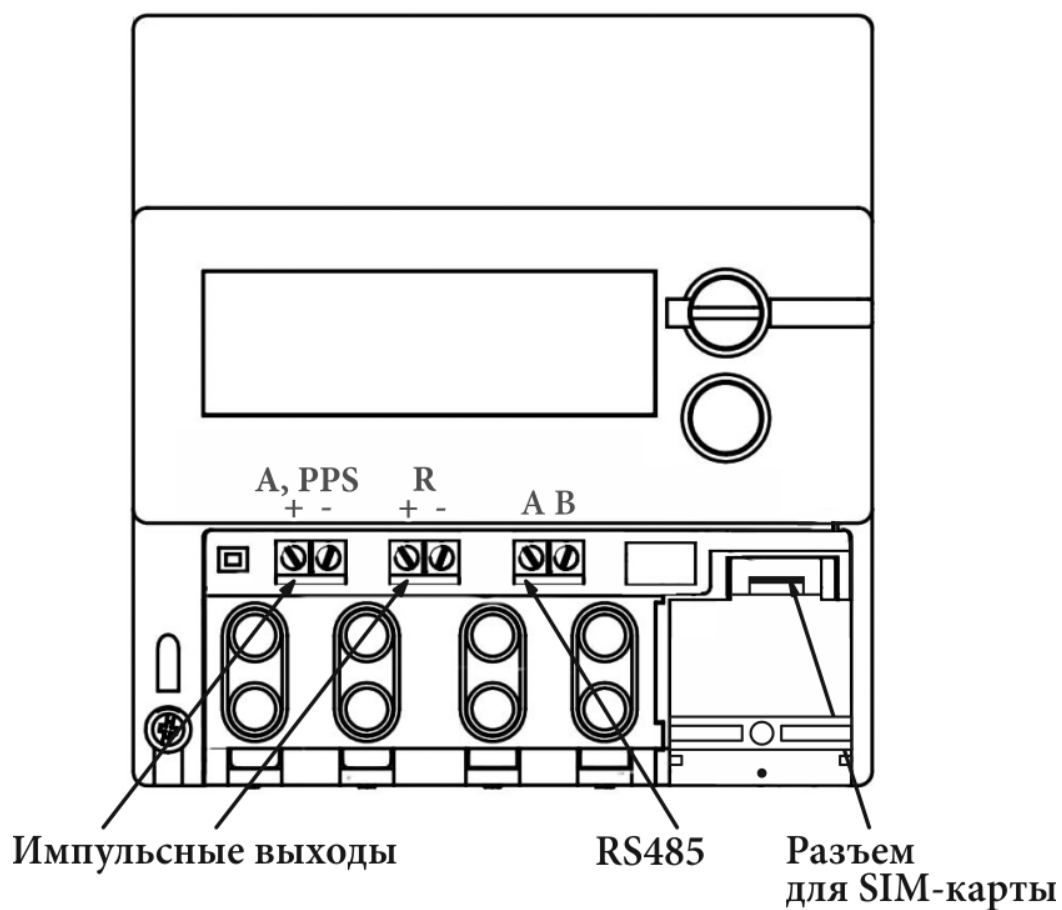
Интерфейсы счетчиков ЛЕ-2 модели D6
