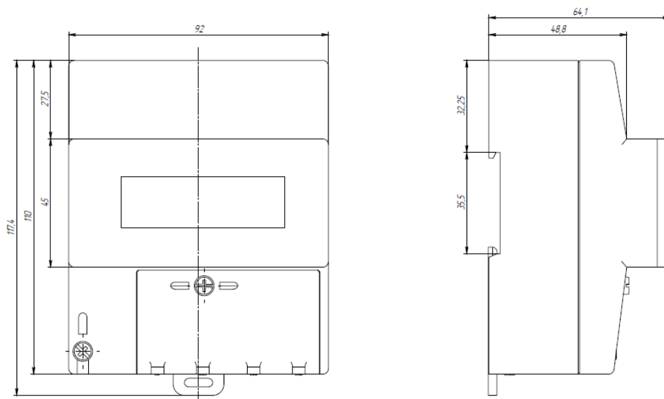
Внешний вид счетчиков ЛЕ-2 моделей D1, D5
