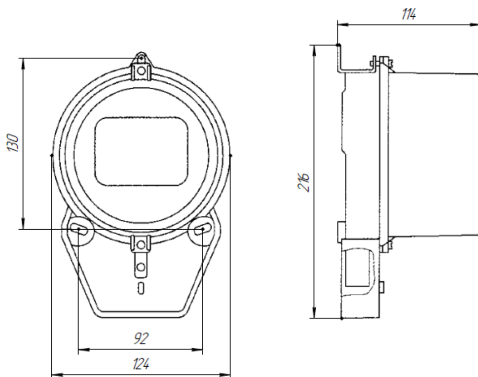
Внешний вид счетчиков ЛЕ-2 моделей P1, P5
