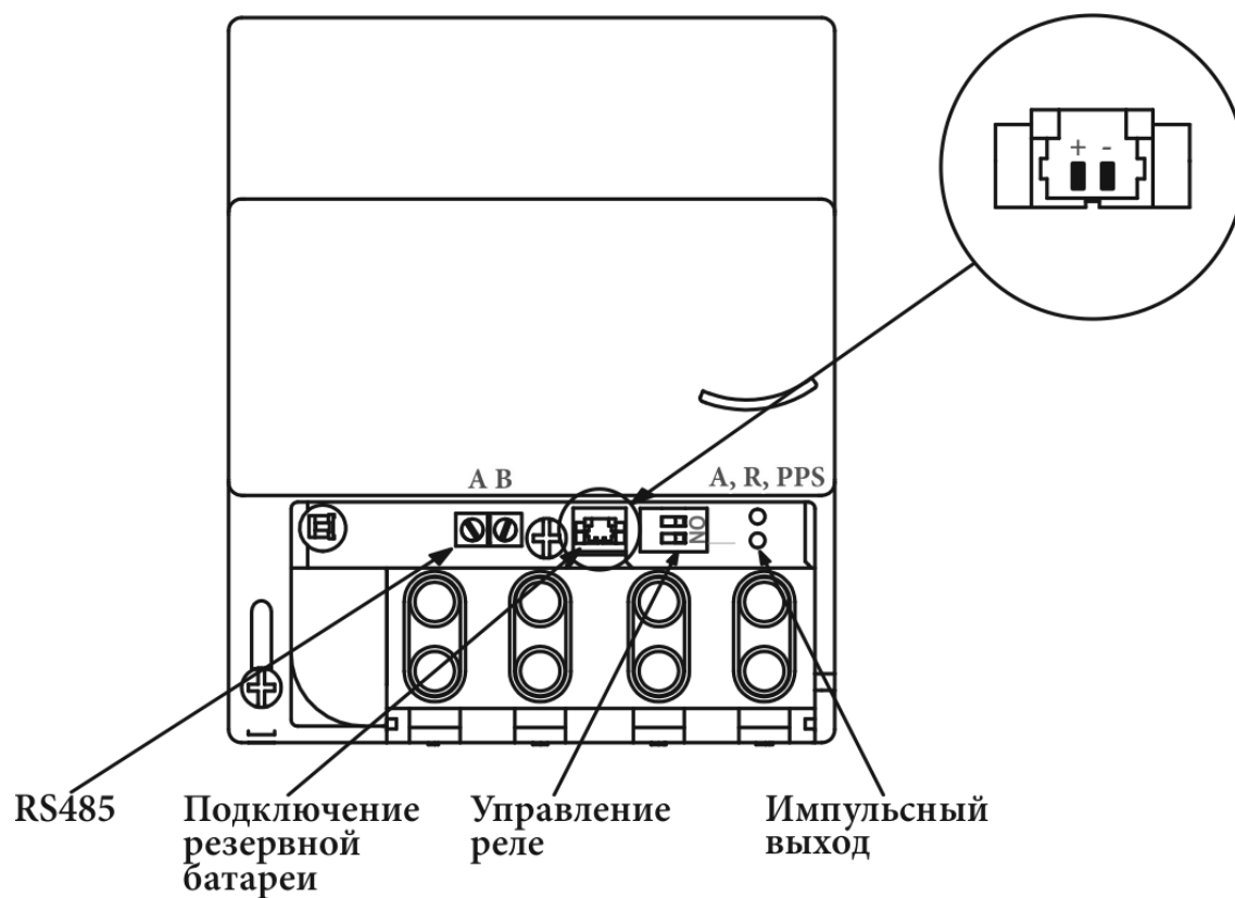
Интерфейсы счетчиков ЛЕ-2 модели D5 с переключателем управления реле
