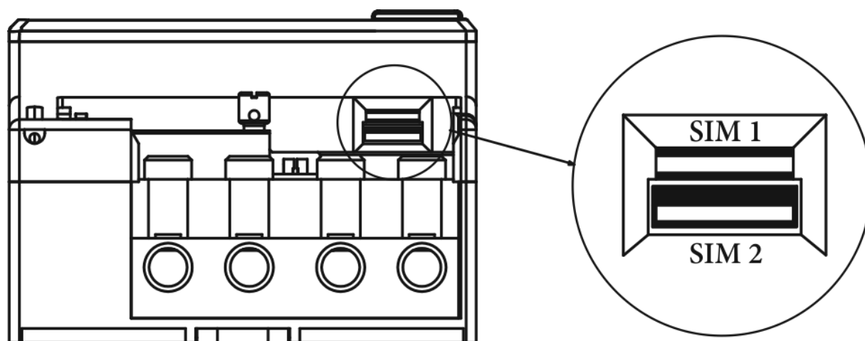
Расположение разъемов для SIM-карт счетчиков ЛЕ-2 модели D5 (вид снизу)
