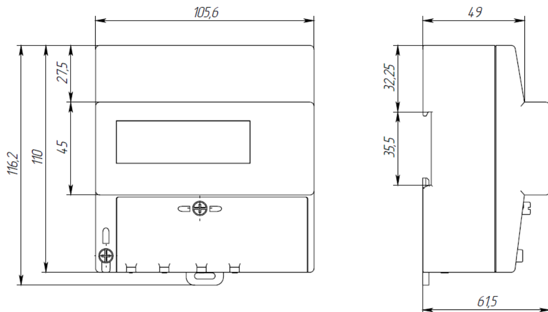
Внешний вид счетчиков ЛЕ-2 моделей D2, D6
